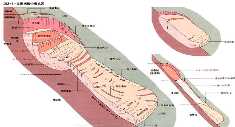
地すべりの模式図
